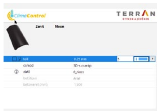
gerincelem
